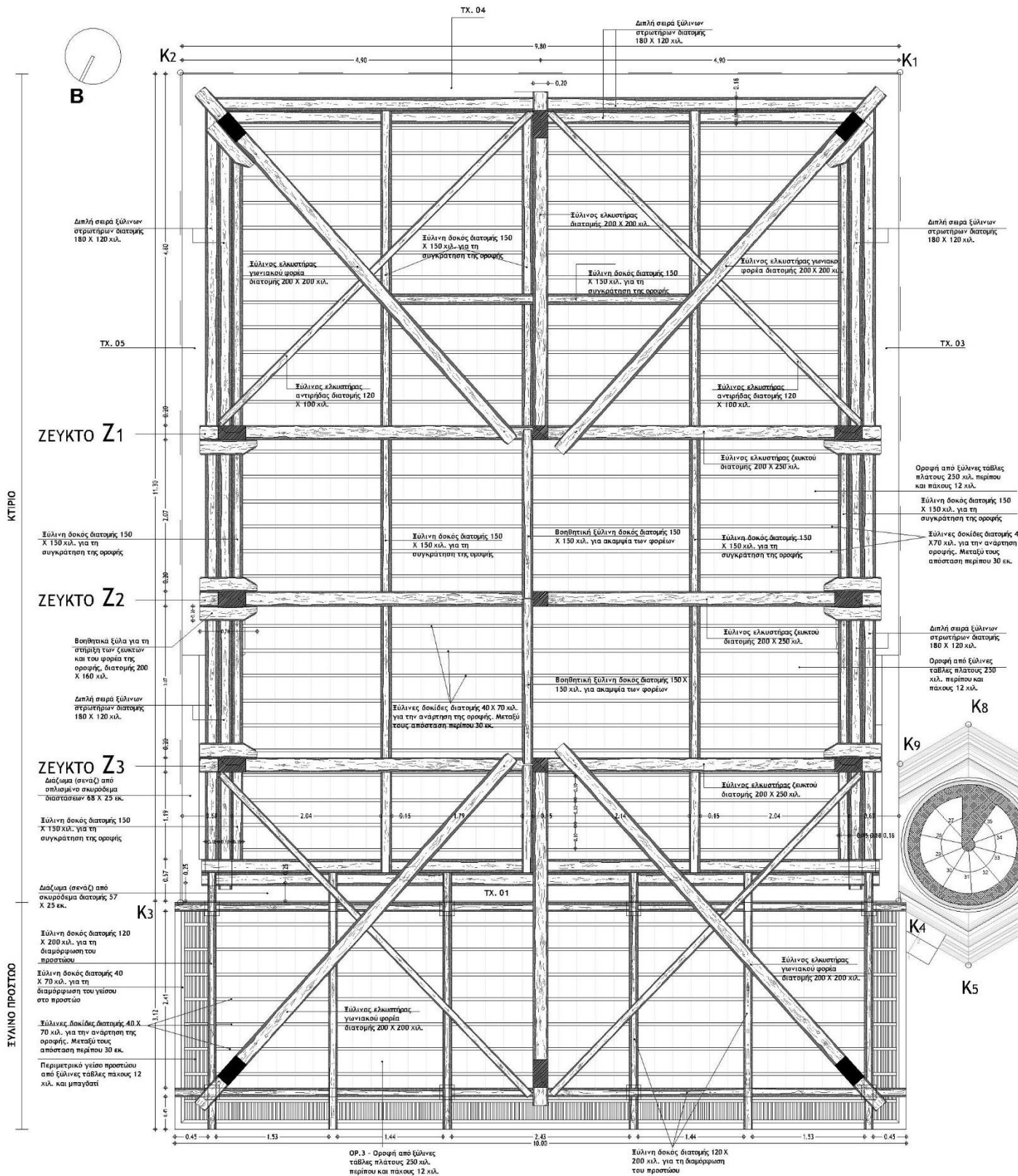
Σχ 1. Κάτοψη οριζοντίων στοιχείων στέγης
