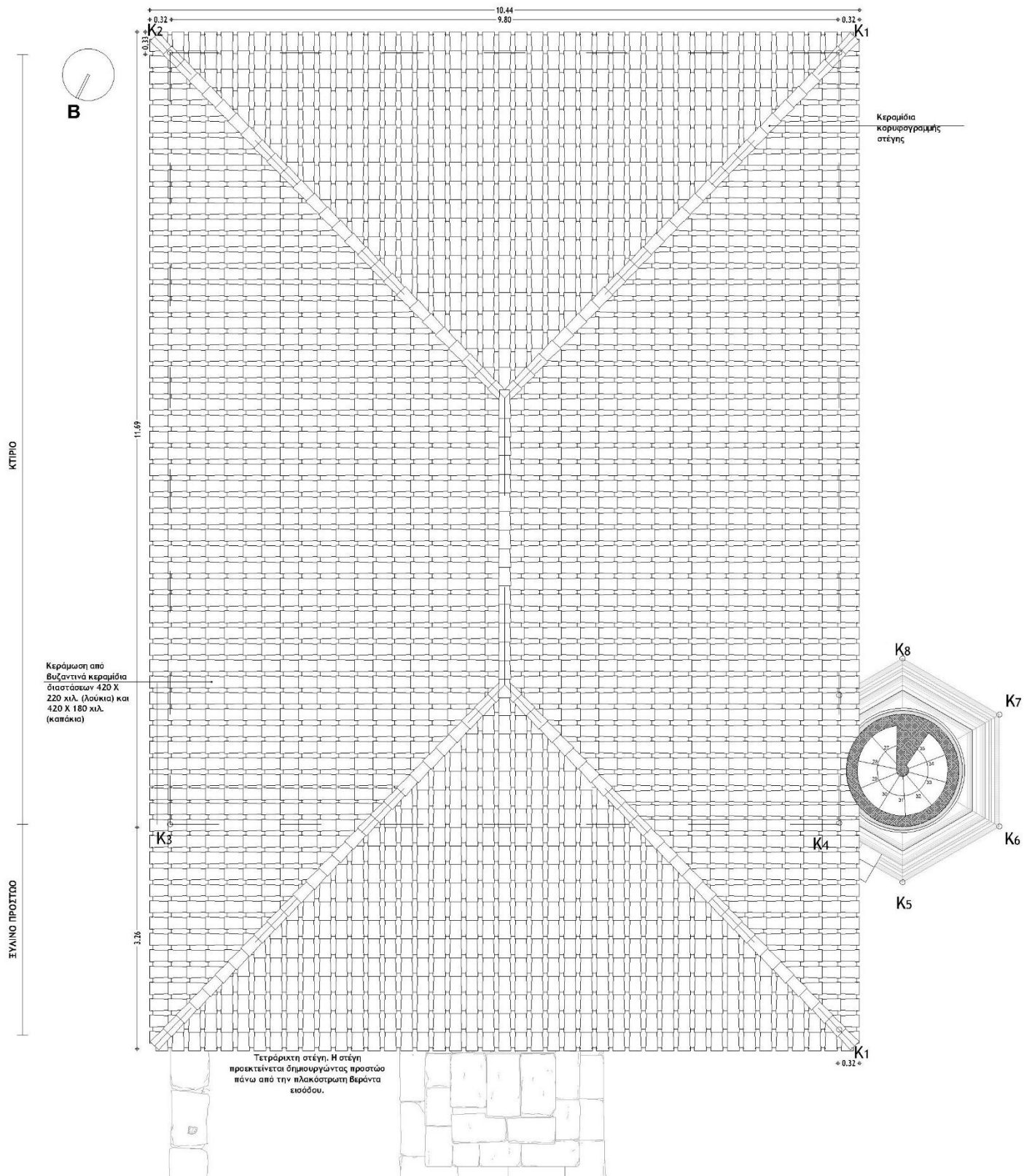
Σχ 3. Κάτοψη κεράμωσης
